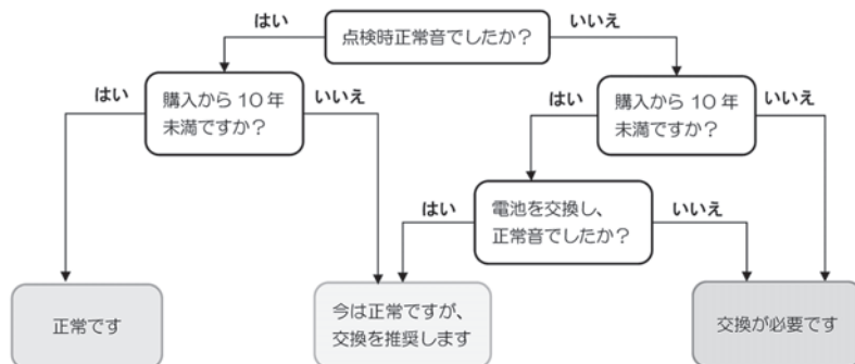
住宅用火災警報器点検フローチャート
